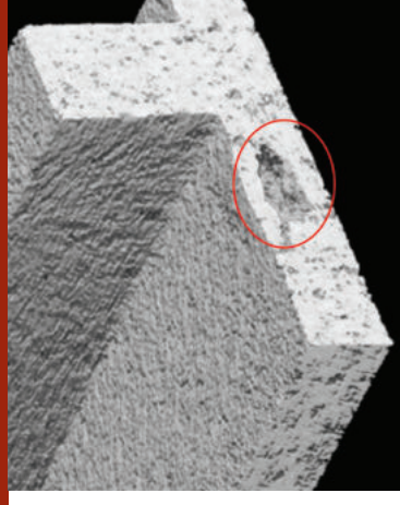
Mikroriss in LDS-Leiterbahn (Rasterelektronenmikroskop)
